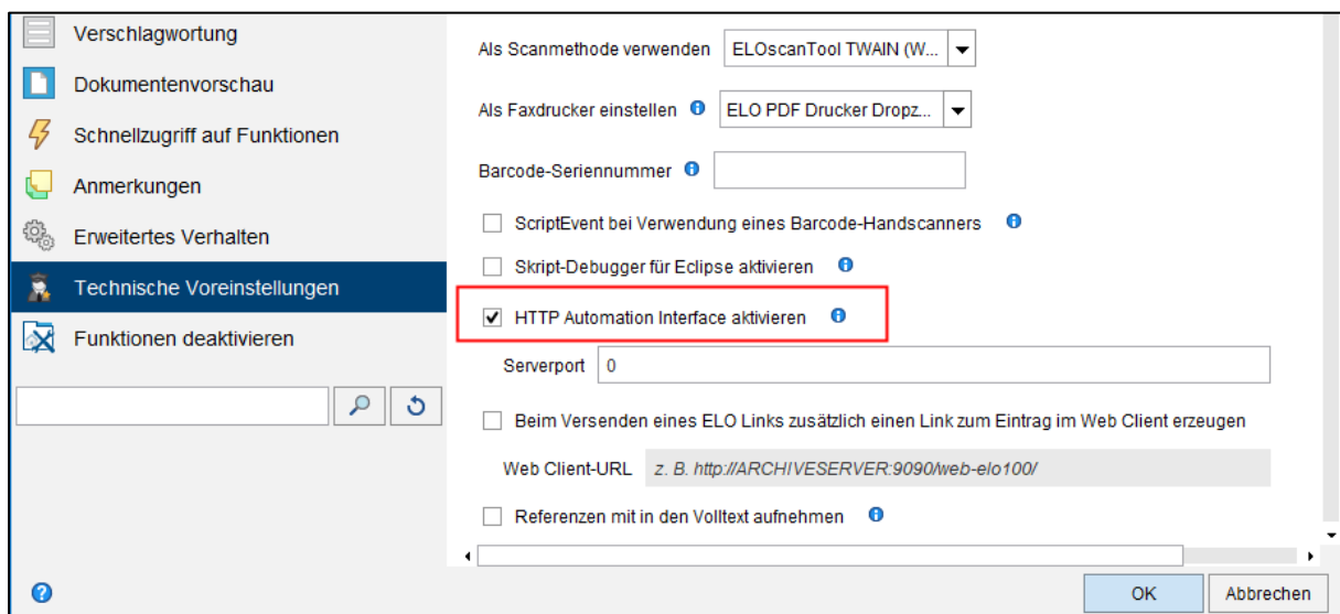
Abb. 1: Konfiguration des ELO Java Clients
